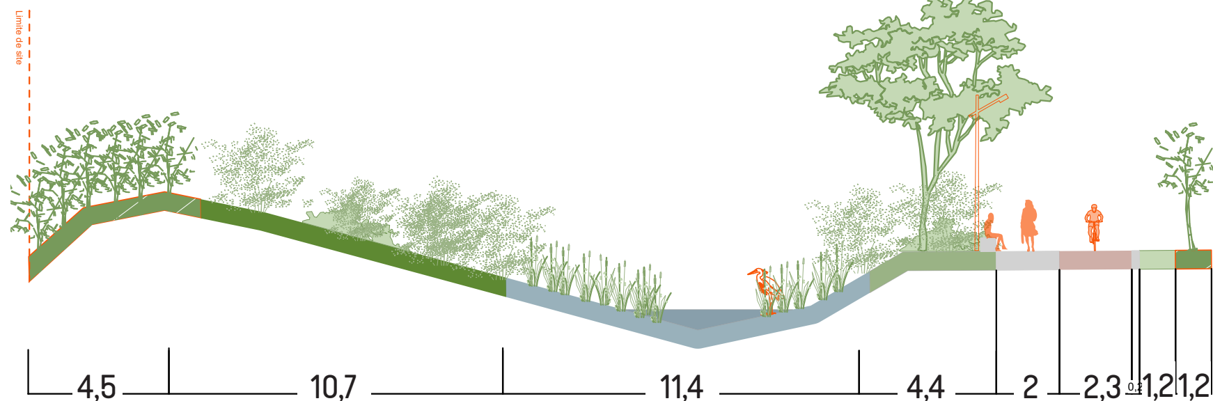
COUPE BB' - LA ZONE HUMIDE AUGMENTÉE
