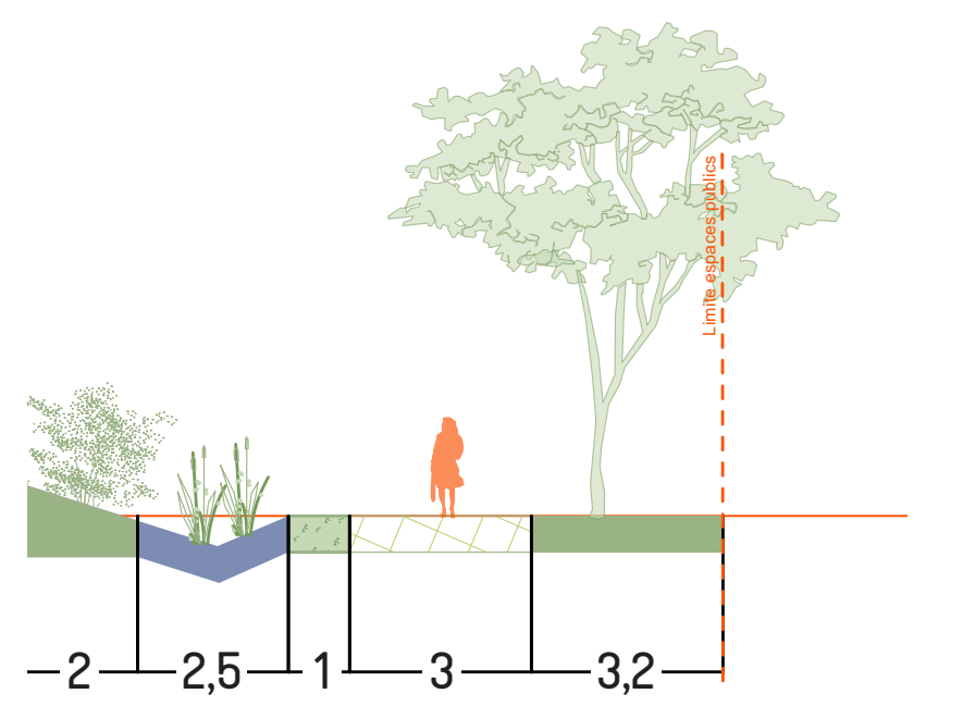
COUPE EE' - LA DRÈVE NORD
