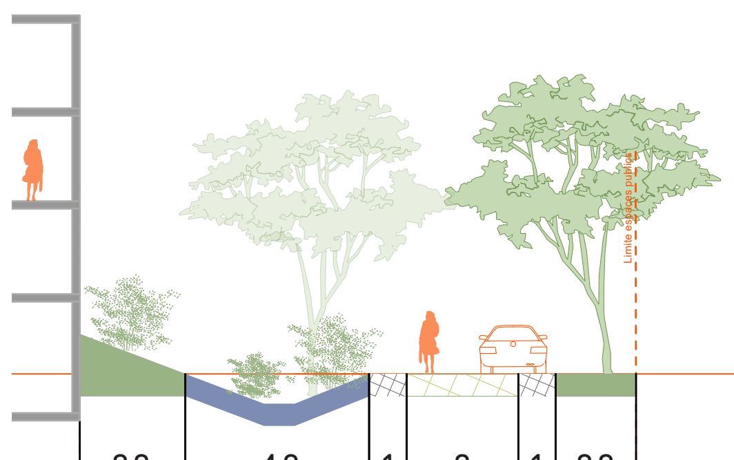
COUPE DD' - LA DRÈVE NORD-EST
